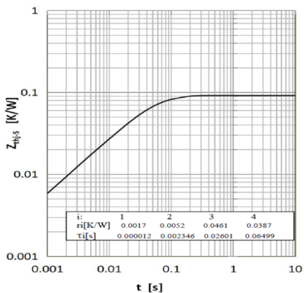
瞬态热阻抗 IGBT, 逆变器 transient thermal impedance IGBT, Inverter
