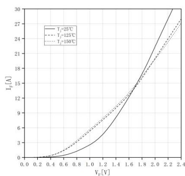
正向偏压特性 二极管, 制动-斩波器 (典型) forward characteristic of Diode, Brake-Chopper (typical)
