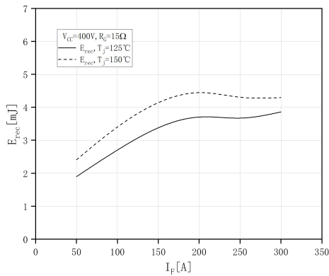
开关损耗二极管(D1, D2, D3, D4), 逆变器 (典型) Switching losses Diode(D1, D2, D3, D4), Inverter(typical)
