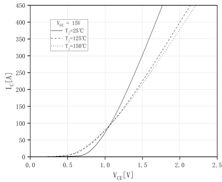
输出特性 IGBT(Q1, Q4), 逆变器 (典型) Output characteristic IGBT(Q1, Q4), Inverter (typical)
