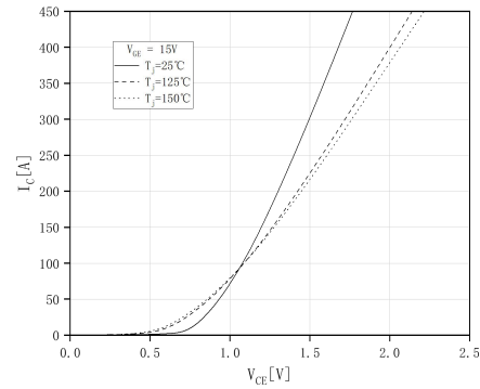
输出特性 IGBT(Q2, Q3), 逆变器 (典型) Output characteristic IGBT(Q2, Q3), Inverter (typical)
