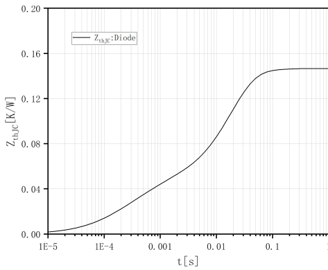
瞬态热阻抗 二极管, D5,D6 Transient thermal impedance Diode
