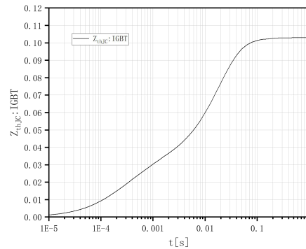
瞬态热阻抗 IGBT(Q2, Q3), 逆变器 Transient thermal impedance IGBT(Q2, Q3), Inverter
