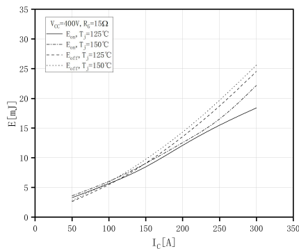
开关损耗 IGBT(Q1, Q4), 逆变器 (典型) Switching losses IGBT(Q1, Q4), Inverter (typical)
