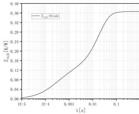
瞬态热阻抗 二极管, D1,D2,D3,D4 Transient thermal impedance Diode
